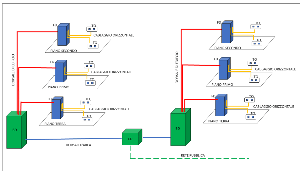
Figura 2 – Esempio di un cablaggio strutturato in un edificio di un comprensorio privato
