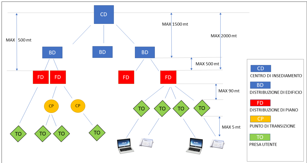
Figura 1 - Struttura e topologia del cablaggio
